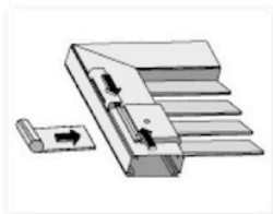
Schematische Darstellung der Funktion von SystemFix
